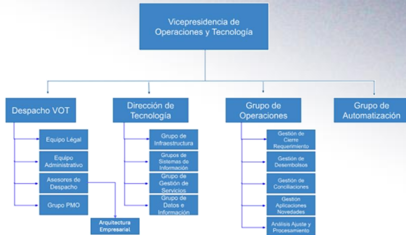
Ilustración 6 Organigrama TI
